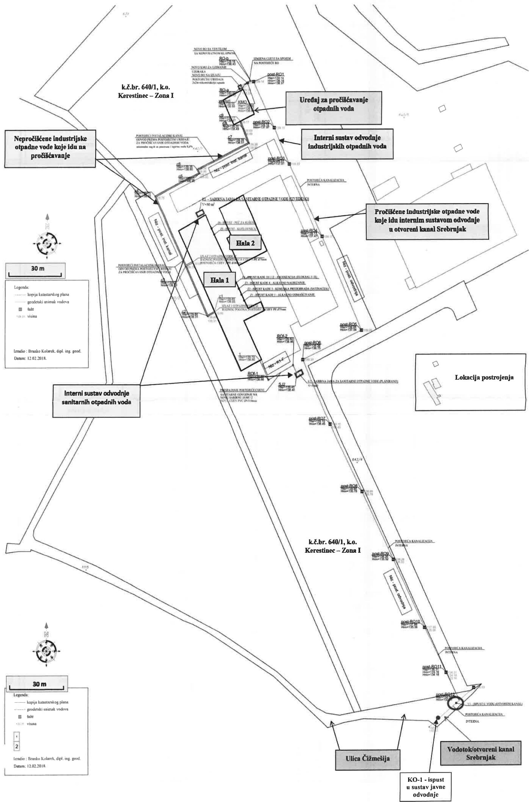
Prilog 3. Situacija sa prikazom objekta, mjesta emisija i dispozicije toka vode na lokaciji postrojenja
