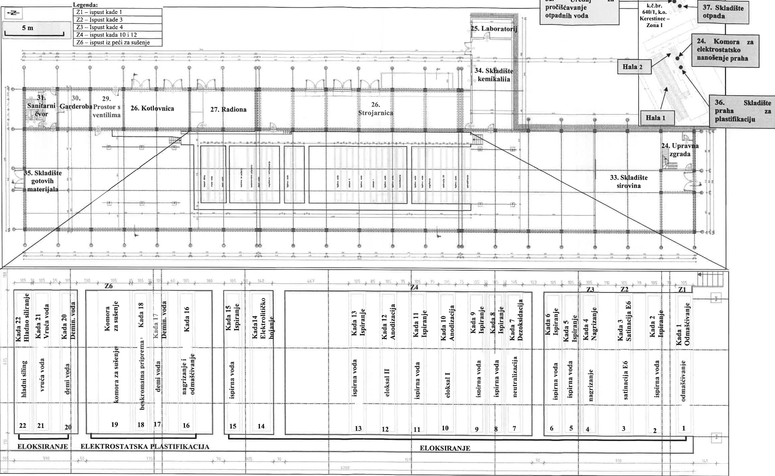
Prilog 2. Situacija sa prikazom objekata na lokaciji postrojenja
